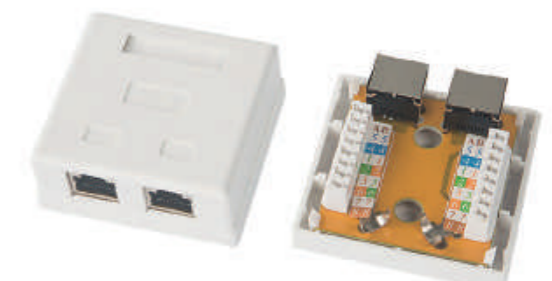
TOM-SB-04-C5E/C6 Surface Box 2 Ports STP Cat5E/CAT6 PCB Jack
